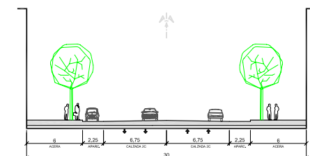
RED VIARIA LOCAL COLECTORA (30 m.) - SECCIÓN 9
