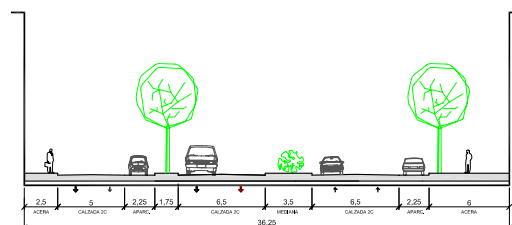
RED VIARIA DISTRITAL (36,25 m.) - SECCIÓN 6'
