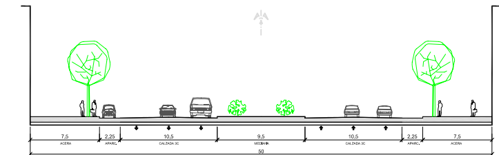
RED VIARIA DISTRITAL (50 m.) - SECCIÓN 2
