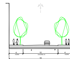
RED LOCAL ACCESO (18 m.) - SECCIÓN 8
