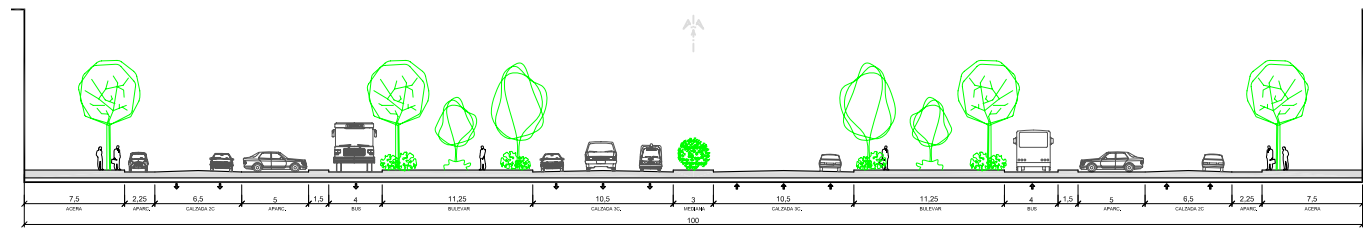
RED VIARIA URBANA (100 m.) - SECCIÓN 1
