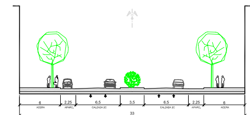
RED VIARIA LOCAL COLECTORA (33 m.) - SECCIÓN 6
