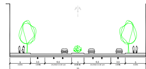
RED VIARIA LOCAL COLECTORA (33 m.) - SECCIÓN 7
