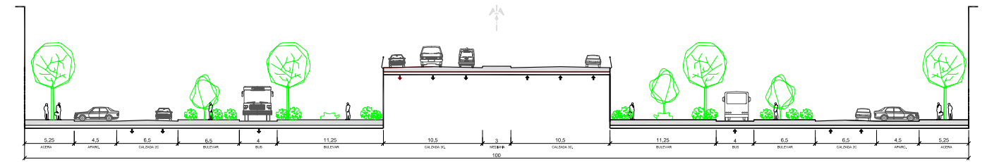
RED VIARIA URBANA (100 m.) - SECCIÓN 1'
