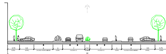
RED VIARIA DISTRITAL (50 m.) - SECCIÓN 4
