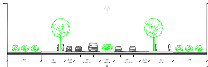
RED VIARIA DISTRITAL (50 m.) - SECCIÓN 3
