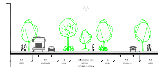
RED VIARIA DISTRITAL (VARIABLE: 50 - 37,73 m.) - SECCIÓN 5
